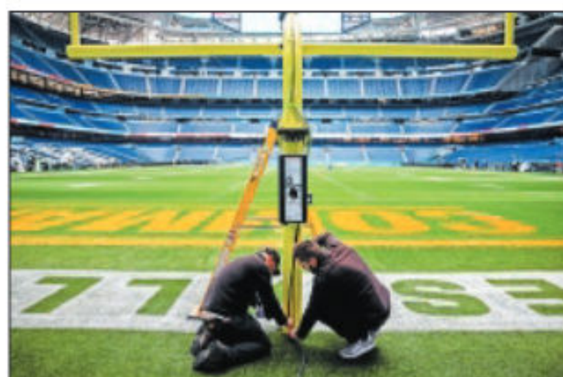
Colocación de los postes en un fondo.
