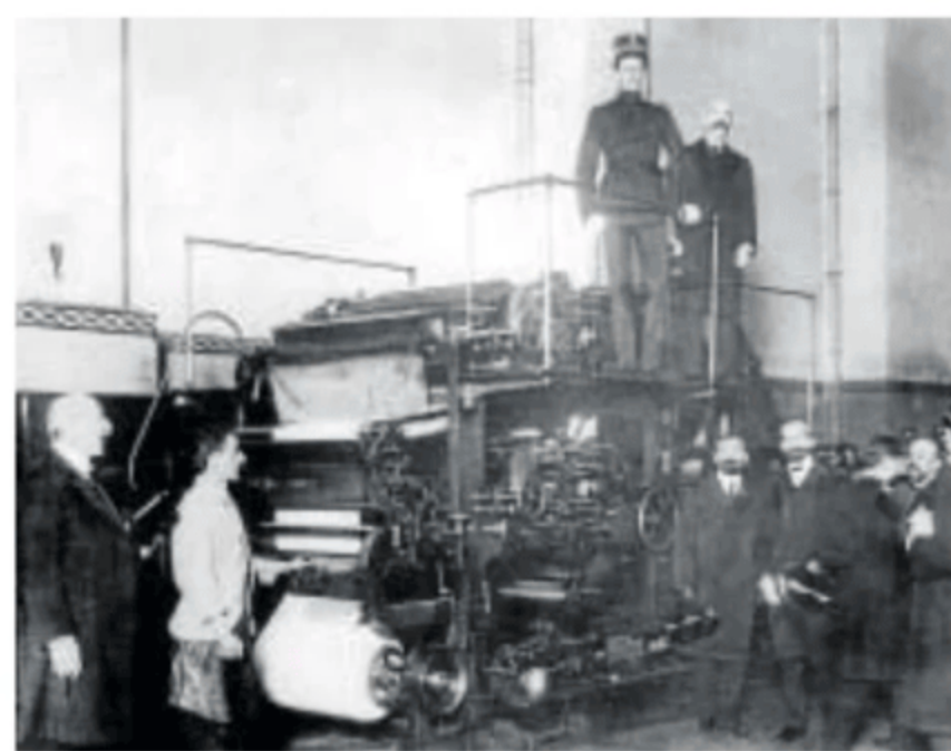
Alfonso XIII, con Torcuato Luca de Tena, en el estribo de una de las cinco rotativas Siemens que ABC adquirió en 1905
